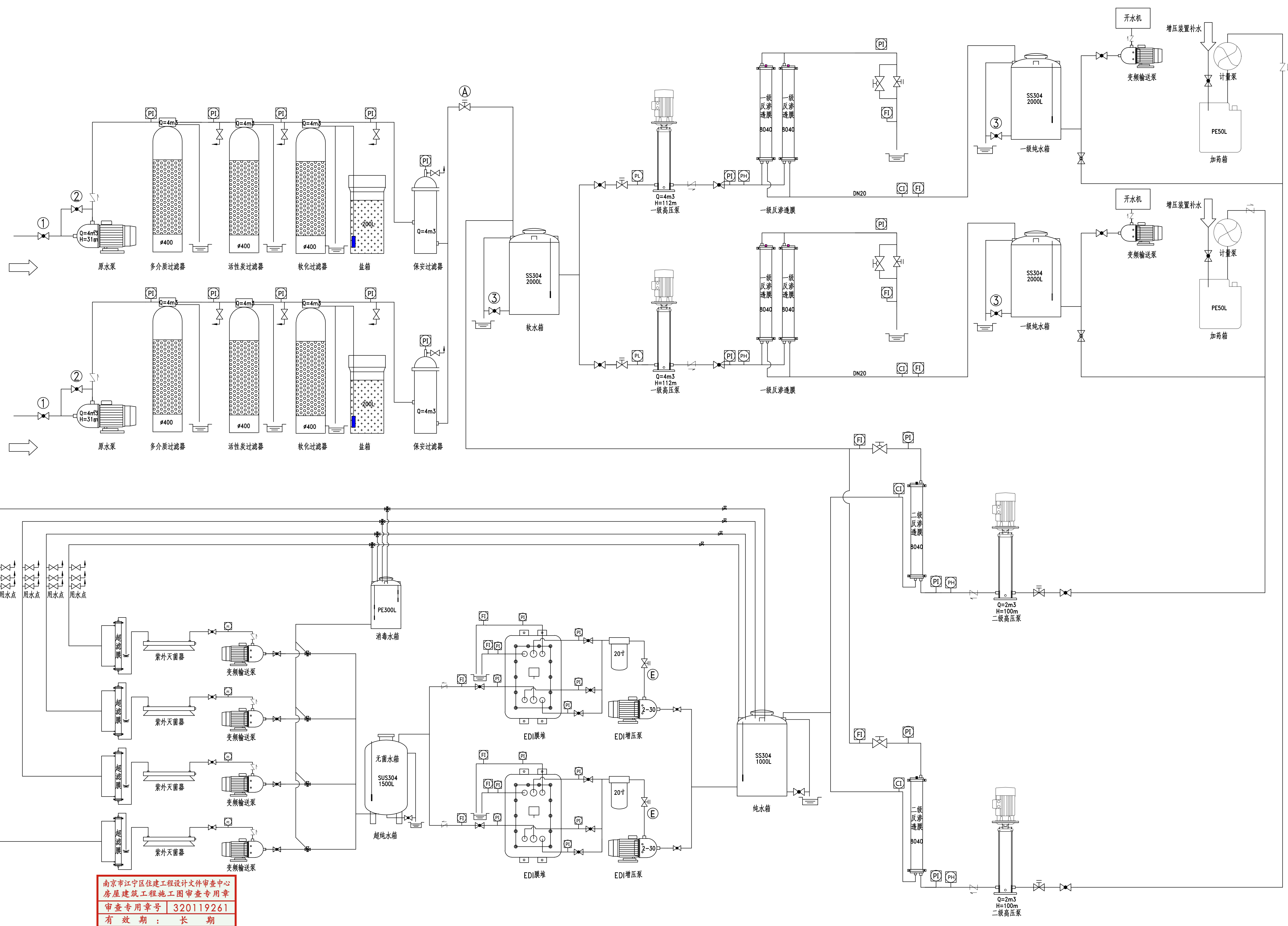
实验室纯水系统流程图
